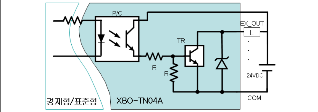
회로구성
