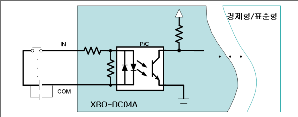
회로 구성
